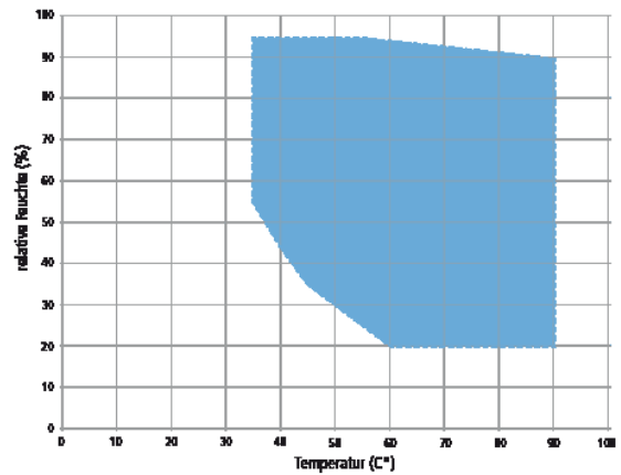
Temperatur-Feuchte-Arbeitsbereich HCP
