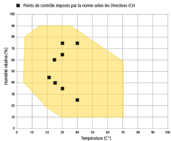
Zone de travail dans la combinaison température – humidité HPP HPP110 - HPP1060 sans lumière
